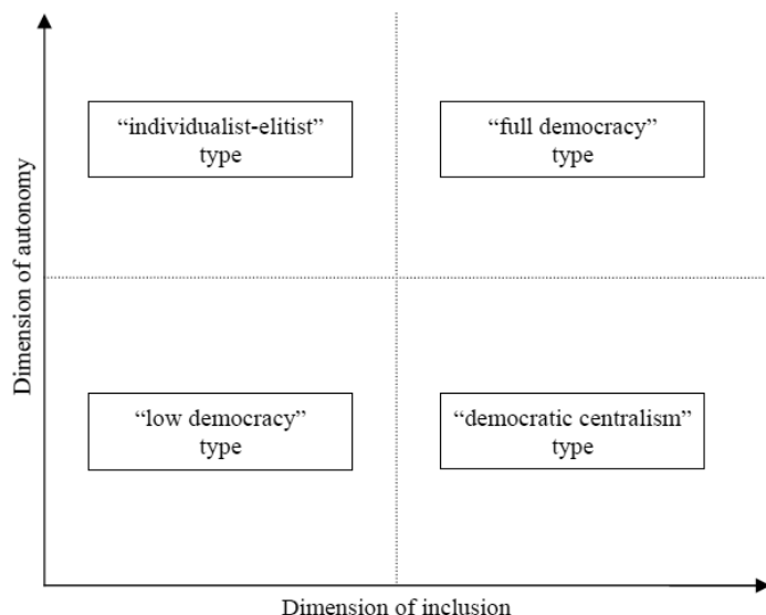
Grafikon 1. Tipovi unutarpartijske demokratije kroz dve dimenzije
