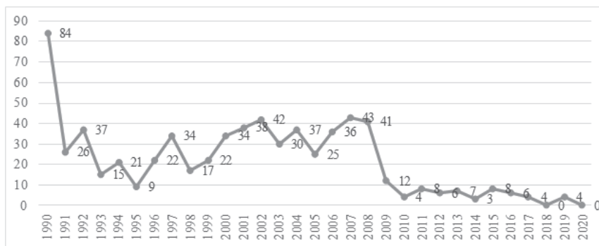
Grafikon 4. Broj novoosnovanih partija od 1990. do 2020. godine (republički i savezni registar)
